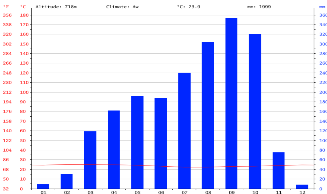
Figure 1. Diagramme ombro-thermique de Makénéné
